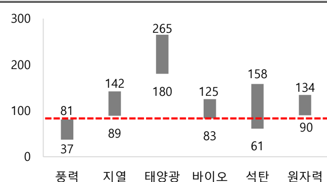
그림 34. 풍력발전의 발전단가 경제성 (단위: $/MWh)
